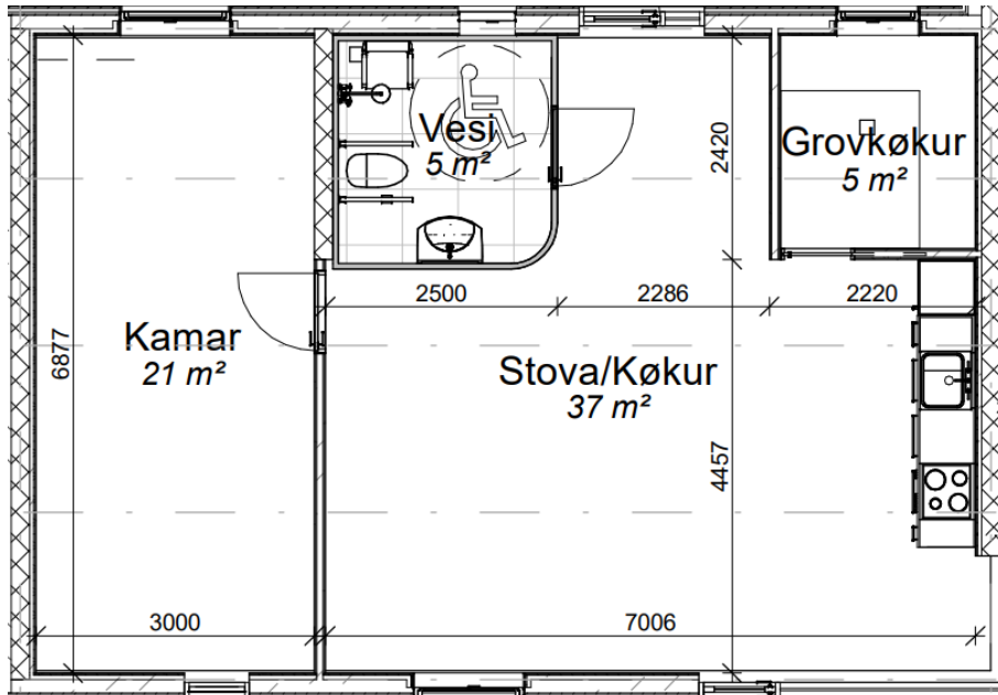
Íbúð 85 m 2 , eignað til fólk við rørslutarni, Óðinshædd 135
