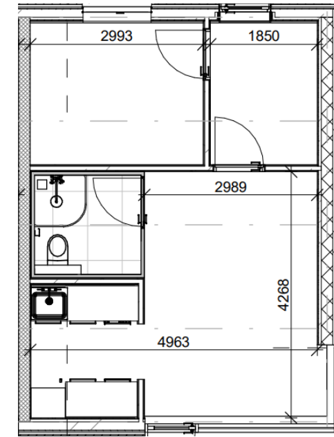
Íbúð 42 m 2 við hornavindeyga, Óðinshædd 141 og 151
